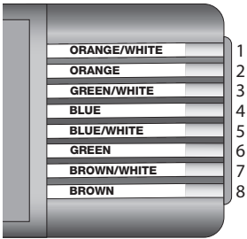
*T-568B wiring
